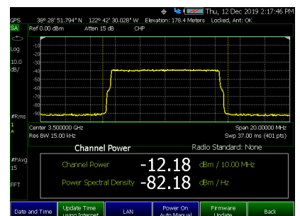
Измерение мощности в канале для сигнала 5G NR FR1
