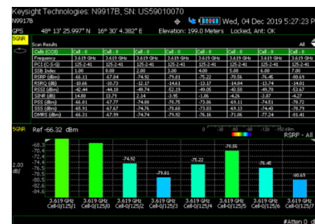
Результаты измерений по радиозфиру каналов управления 5G NR с отображением идентификаторов сот
